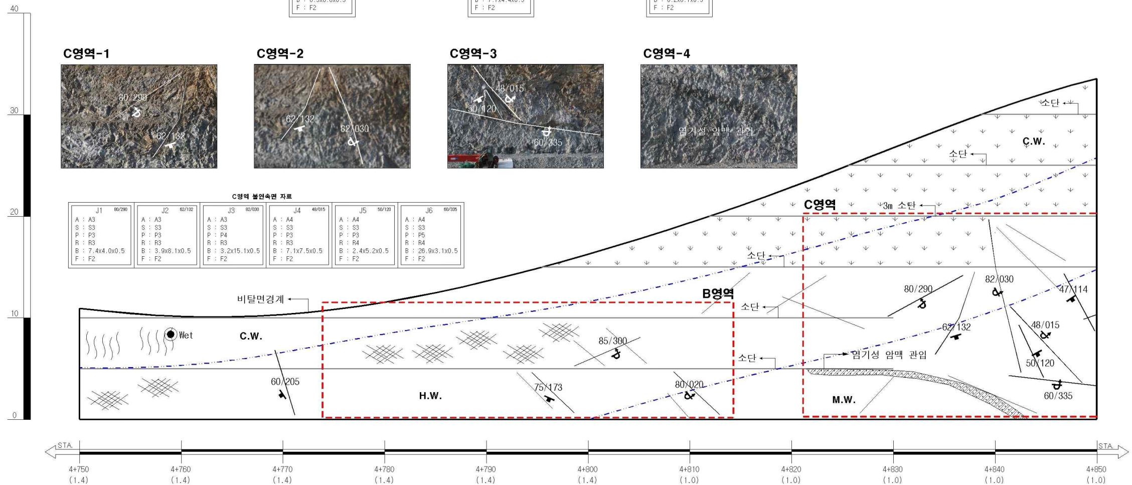
<A-A'단면>
