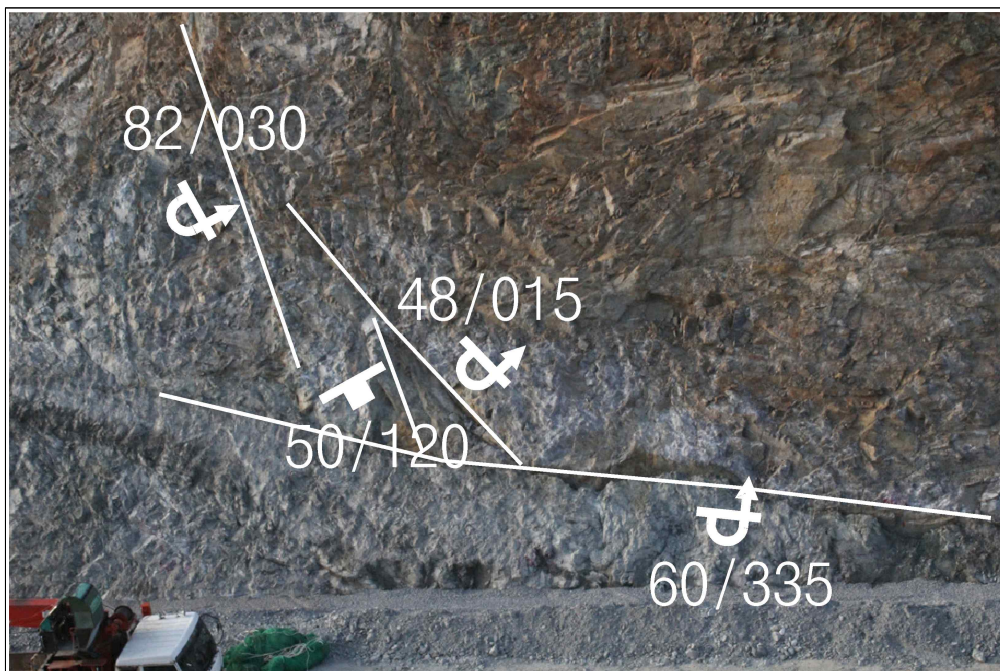
【그림 22】 C 영역에 발달한 불연속면
