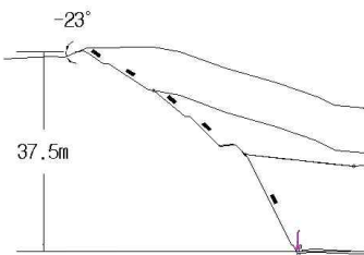
<A-A'단면>
